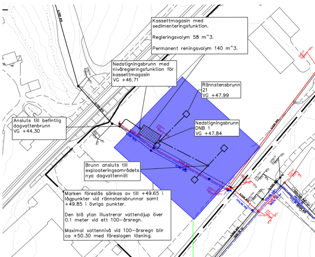
Bild 19: Dagvatten- och skyfallsåtgärder förläggs huvudsakligen till den sydvästra delen av området. (Ur dagvattenutredning av Dämningsverket).
